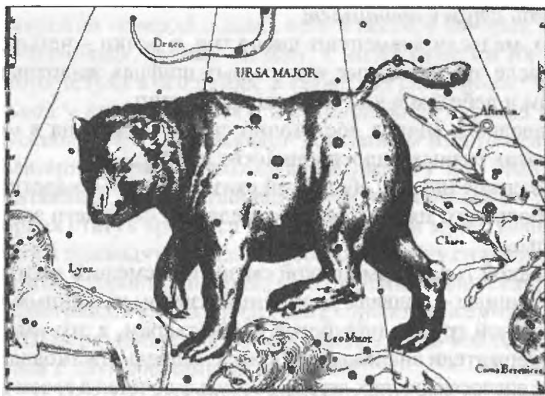
( «Uranografia», 1690)
