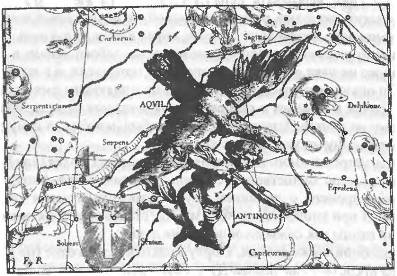
( «Uranografia», 1690)
